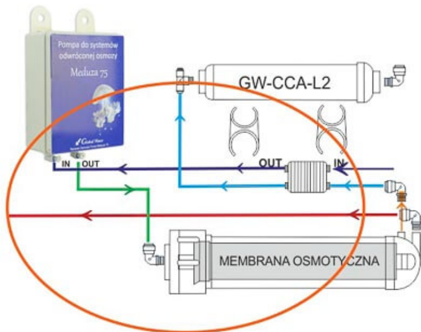
Schemat instalacji pompy w standardowym systemie odwróconej osmozy:
