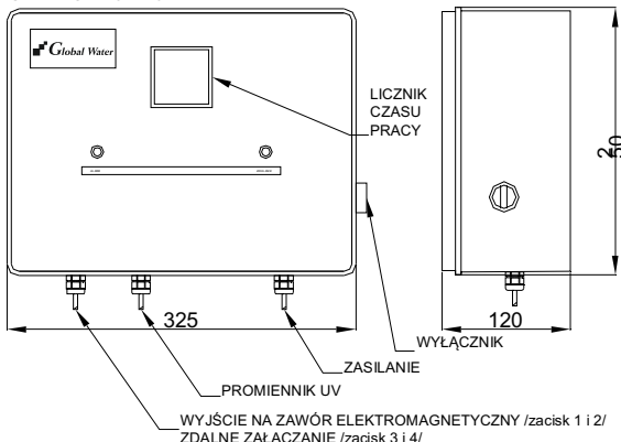
SZAFKA STEROWNICZA
